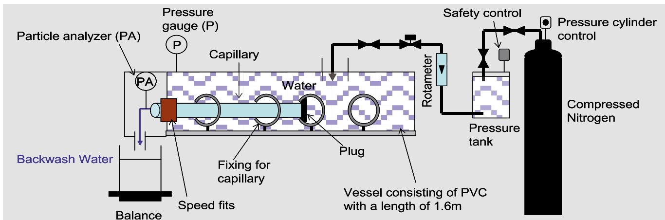
Schematische Darstellung einer Rückspüleinrichtung
